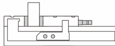
Zuganker-System entspannt
