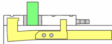
Zuganker-System gespannt
